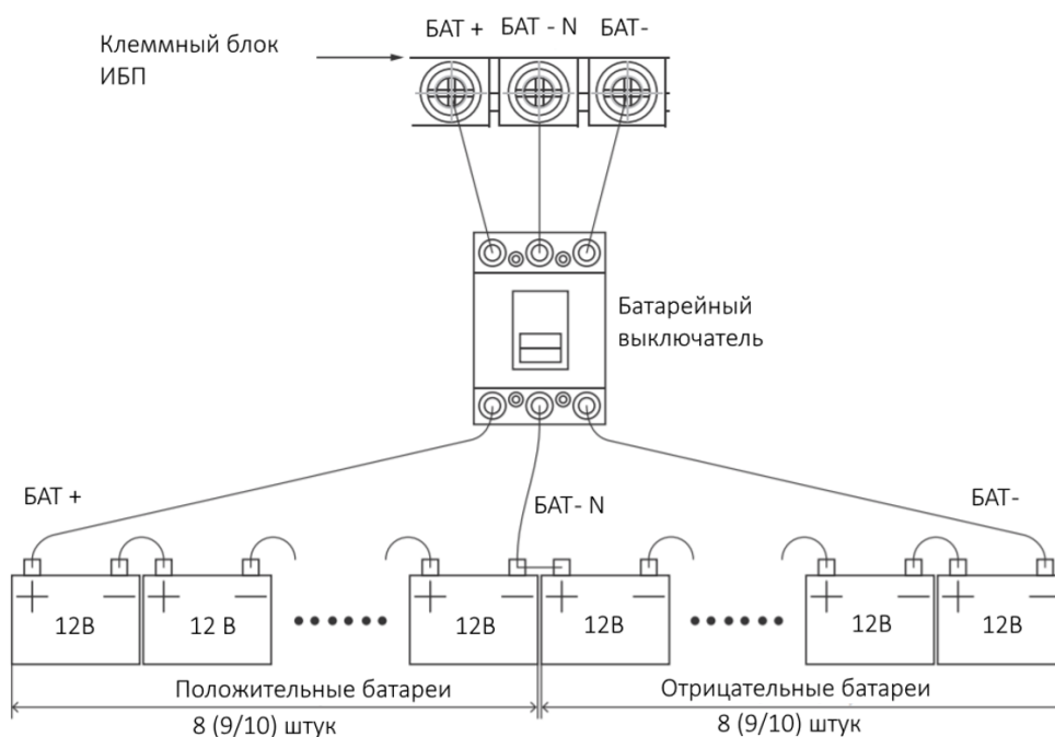
Рис. 3-4 Подключение АКБ
